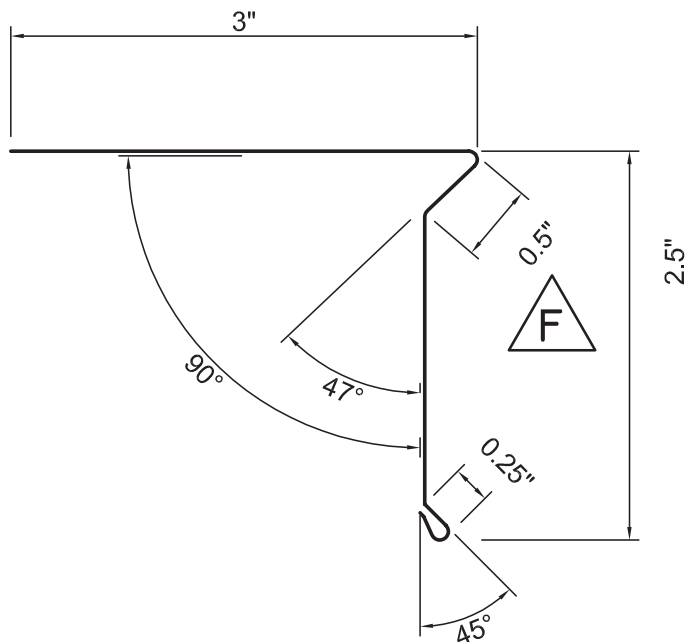
FT02 6" T-STYLE DRIP EDGE
